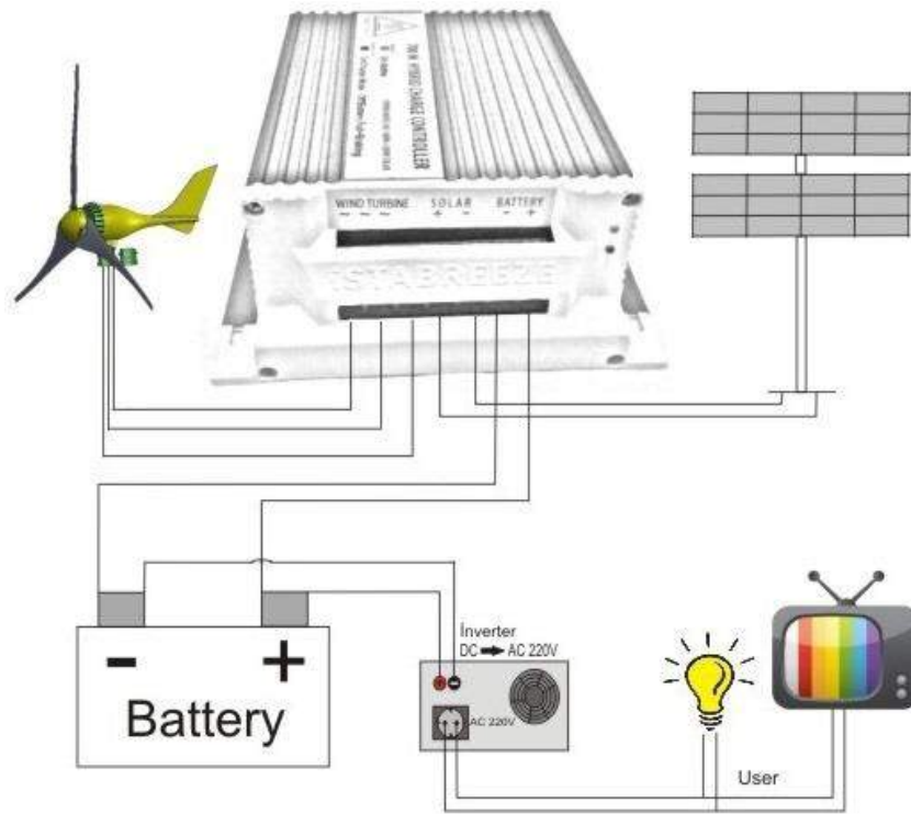
Örnek bağlantı şeması
