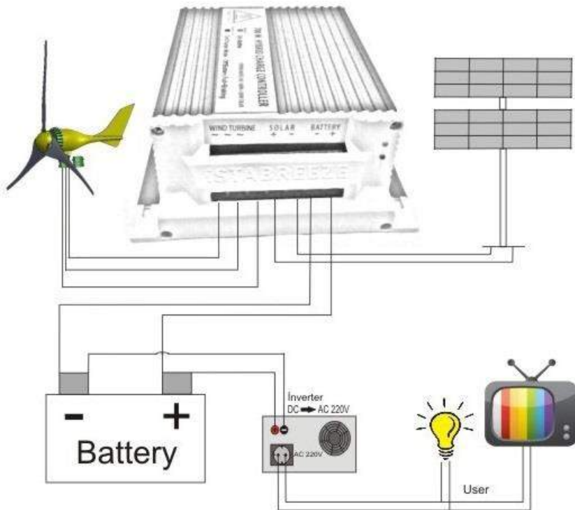
Schaltplan Beispiel
