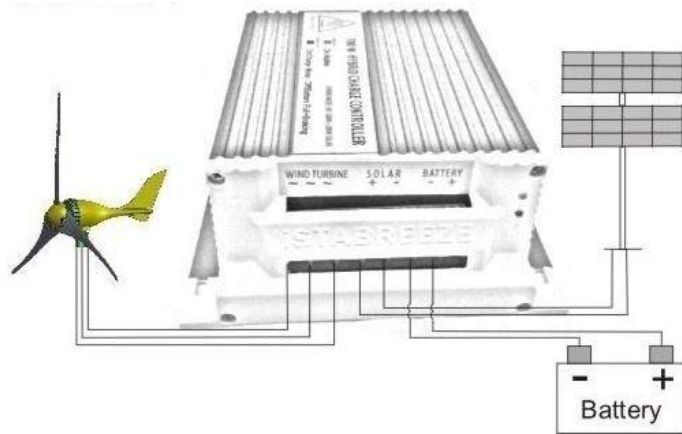
Batterie - und Turbineninstallation mit Controller
